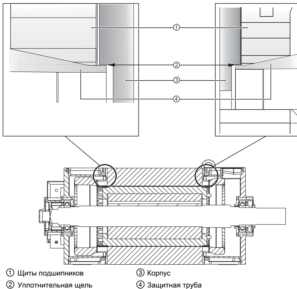
Рис. 9-2 Уплотнительные зазоры между корпусом и щитами подшипников (принципиальная схема)
