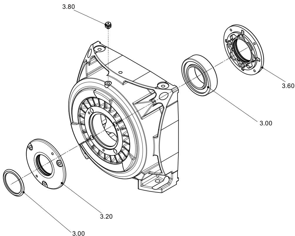
Рис. 11-3 Узел подшипника качения приводная сторона, ременной привод, с дополнительной смазкой
