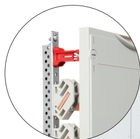
ED-профиль до 400 А
