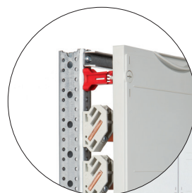
WR-профиль до 850 А
