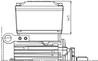
Двигатели типоразмеров 80-132
