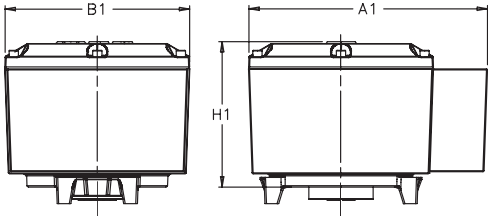
Двигатели типоразмеров 280-315
