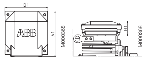
Двигатели типоразмеров 280 - 315
