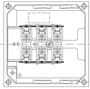
Кабельные зажимы для двигателей типоразмеров 90-112
