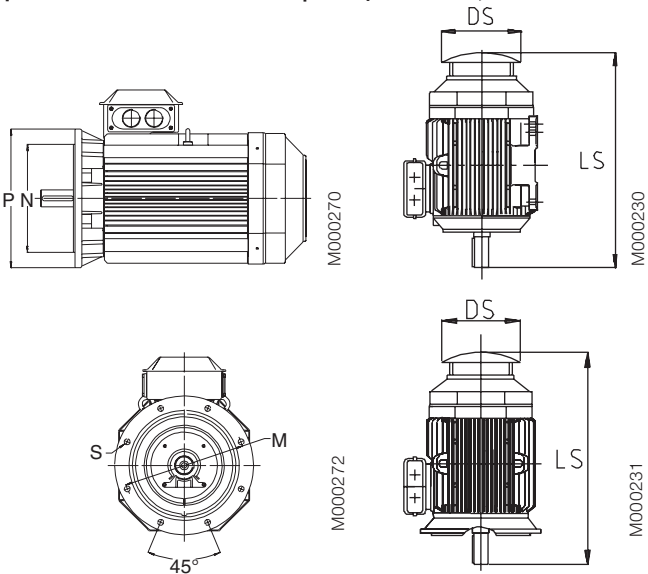
Типоразмеры 225-400
