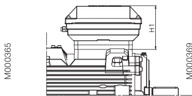
Двигатели типоразмеров 355 - 400
