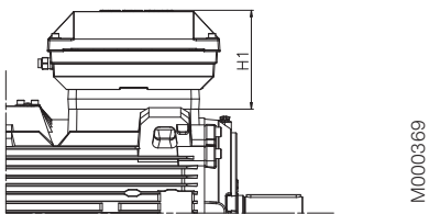
Двигатели типоразмеров 200 - 250
