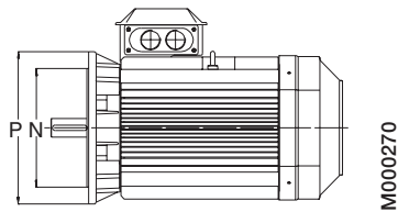
Двигатель с монтажом на фланце IM 3001, IM B5
