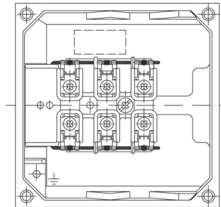
Кабельные зажимы для двигателей типоразмеров 90-112
