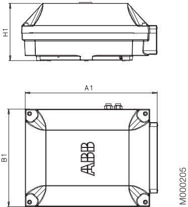
Двигатели типоразмеров 280 - 315
