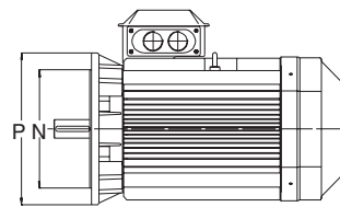
Типоразмеры 225-250
