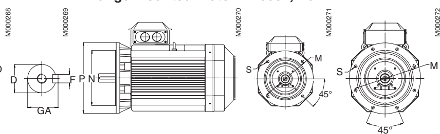
Flange mounted motor IM 3001, B5
