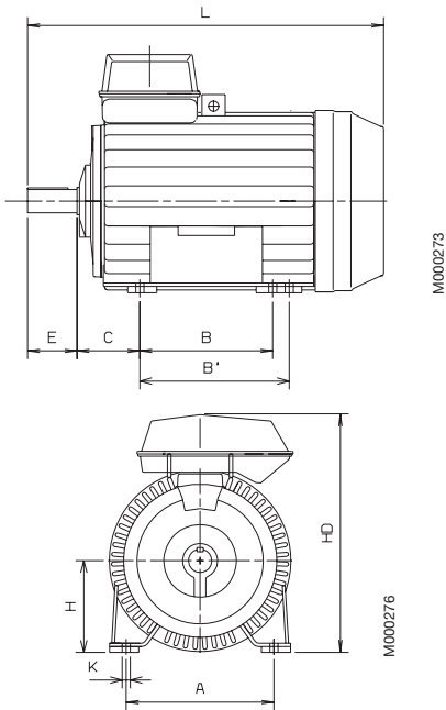
Foot mounted motor IM 1001, B3
