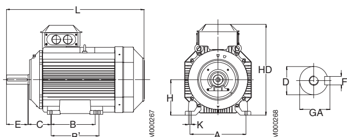
Foot mounted motor IM 1001, B3
