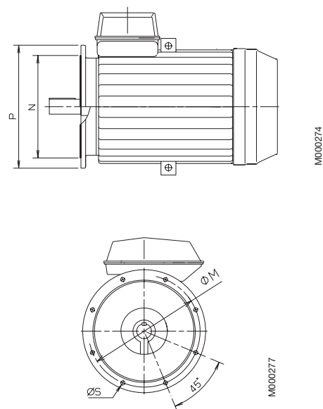
Flange mounted motor IM 3001, B5
