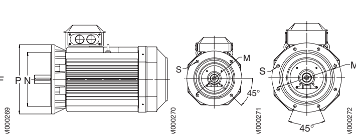
Flange mounted motor IM 3001, B5
