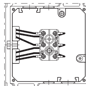
Terminal box size 112-132.
