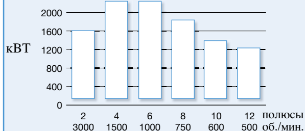
Мощность двигателя HXR при 4000 В 50 Гц
