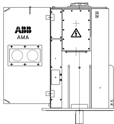
Code I: IM V1 Code II: IM 4011 Vertical flange mounted (free shaft end facing downwards)
