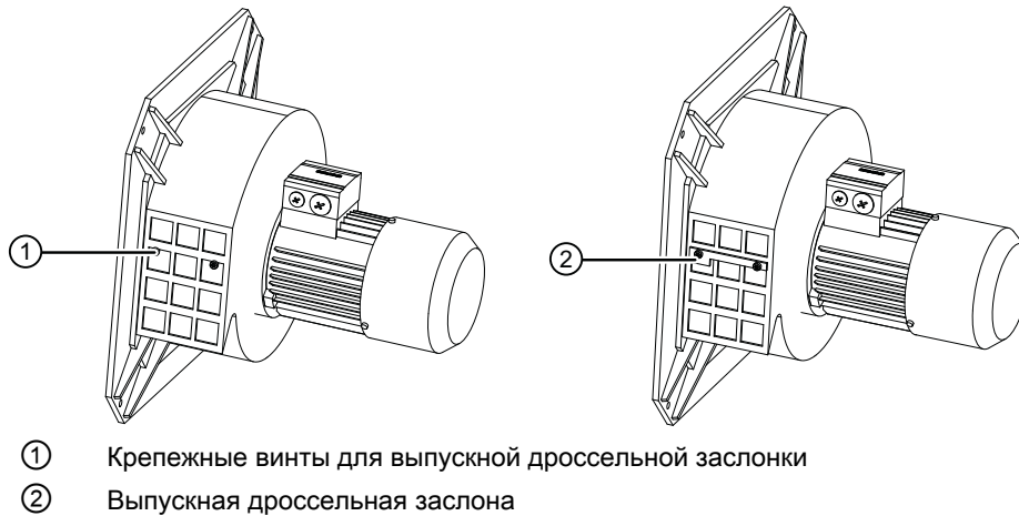
Рис. 6-3 Дроссельная заслонка при всасывающей вентиляции (приводная сторона к неприводной)
