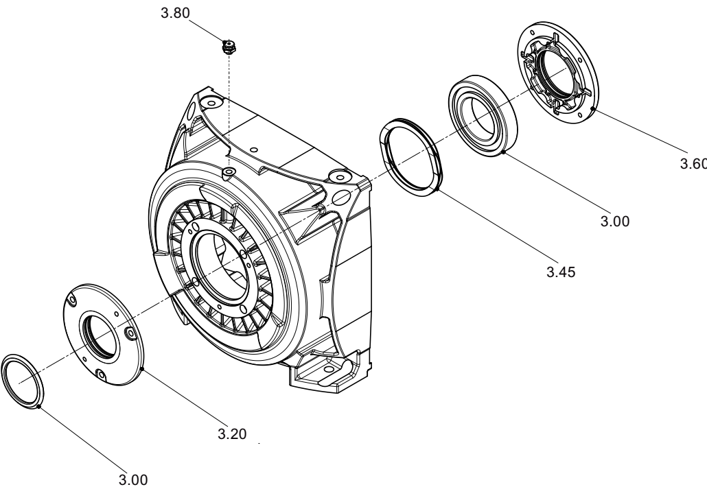
Рис. 11-4 Узел подшипника качения приводная сторона, с приводной муфтой, с дополнительной смазкой
