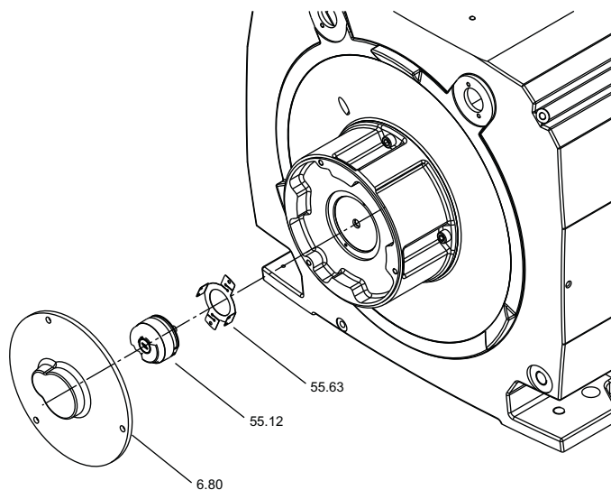
Рис. 11-11 Датчик частоты вращения (тип 1PH828.)
