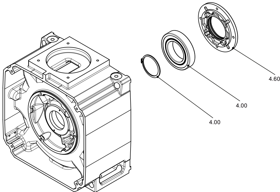
Рис. 11-6 Узел подшипника качения неприводная сторона, непрерывная смазка
