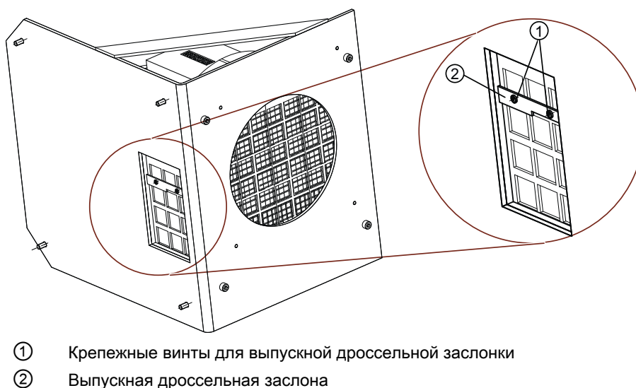
Рис. 6-4 Дроссельная заслонка при нагнетательной вентиляции (неприводная сторона к приводной)
